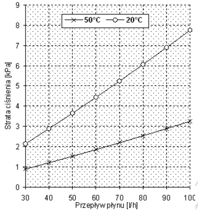
Zależność straty ciśnienia kolektora TS 400 na przepływie cieplonośnego płynu Solaren-Eko
